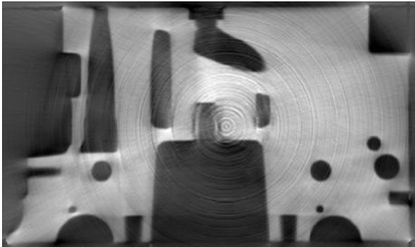
Figuur 2 Ringvormige artefacten in een CT-scan van een VW-cilinderkop
